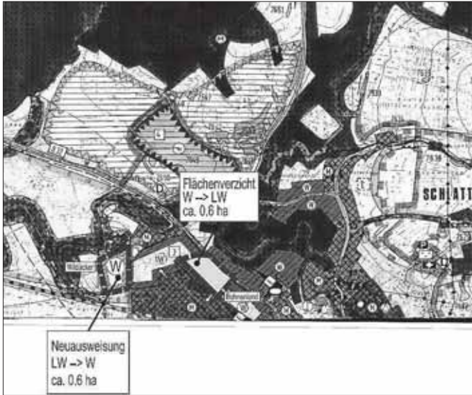
Lageplan Bestand und Planung, Büro Gfrörer, Empfingen, vom 24.05.2018
